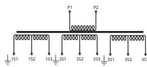
Loại 3 lõi, 2 tỷ số (3 cores, 2 ratios type)
