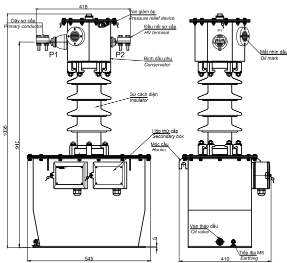
Loại 3 lõi, 2 tỷ số (3 cores, 2 ratios type)
