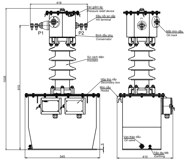
Loại 3 lõi, 3 tỷ số (3 cores, 3 ratios type)
