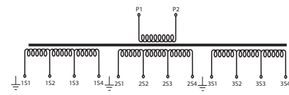
Loại 3 lõi, 3 tỷ số (3 cores, 3 ratios type)
