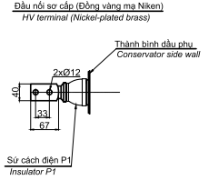
Dòng sơ cấp I_1 ; 300 < I_1 \leq 400A (Primary current I_1 ; 300 < I_1 \leq 400A )
