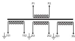
Loại 3 lõi, 1 tỷ số (3 cores, 1 ratio type)
