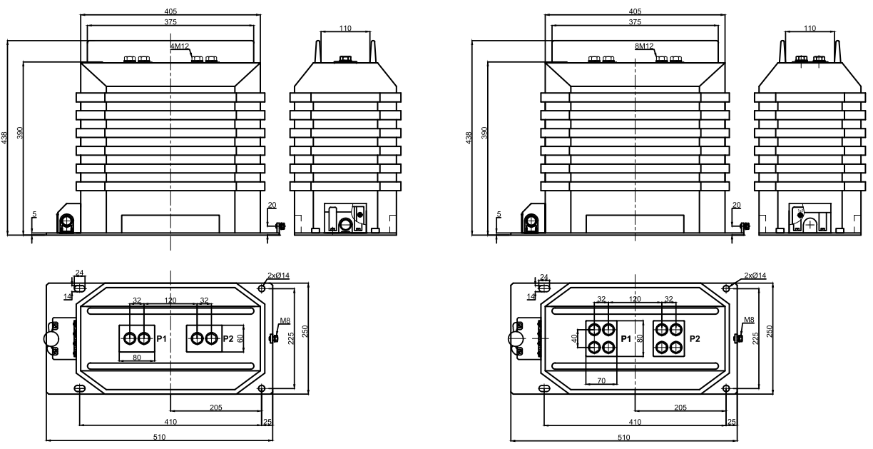
Loại 1: 1 < I_n \leq 1250A
